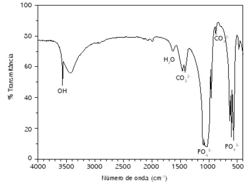
Figura 2: Espectroscopia no infravermelho do pó de hidroxiapatita.
