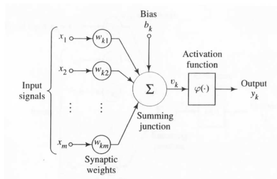
Figura 1: Modelo não-linear de um neurônio k
